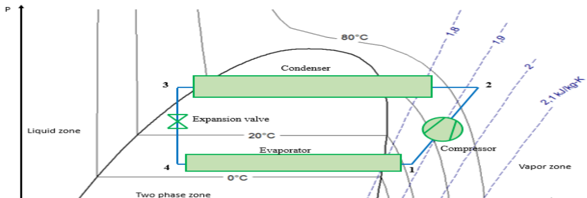
Fig. 3. Vapour compression cycle
