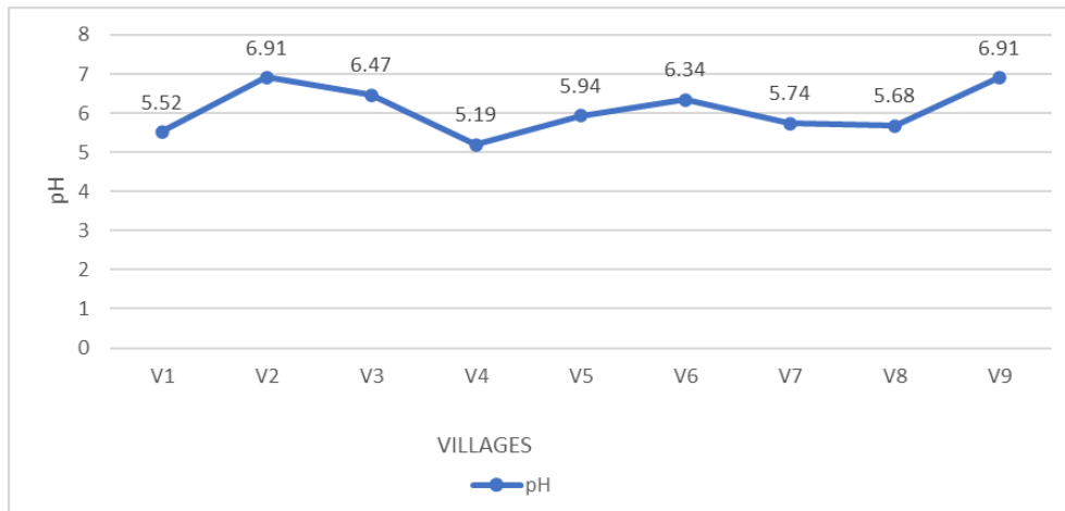
Fig. 3. pH
